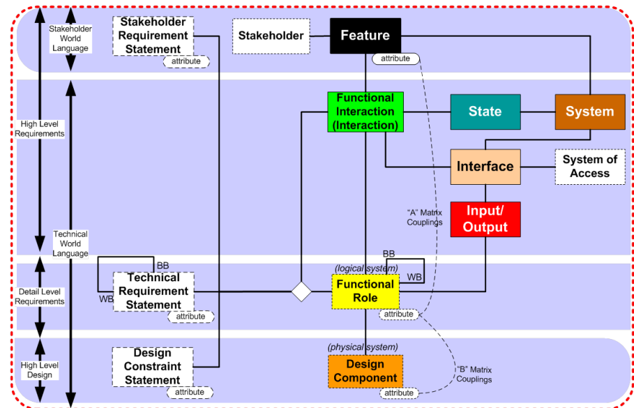
S* Metamodel
